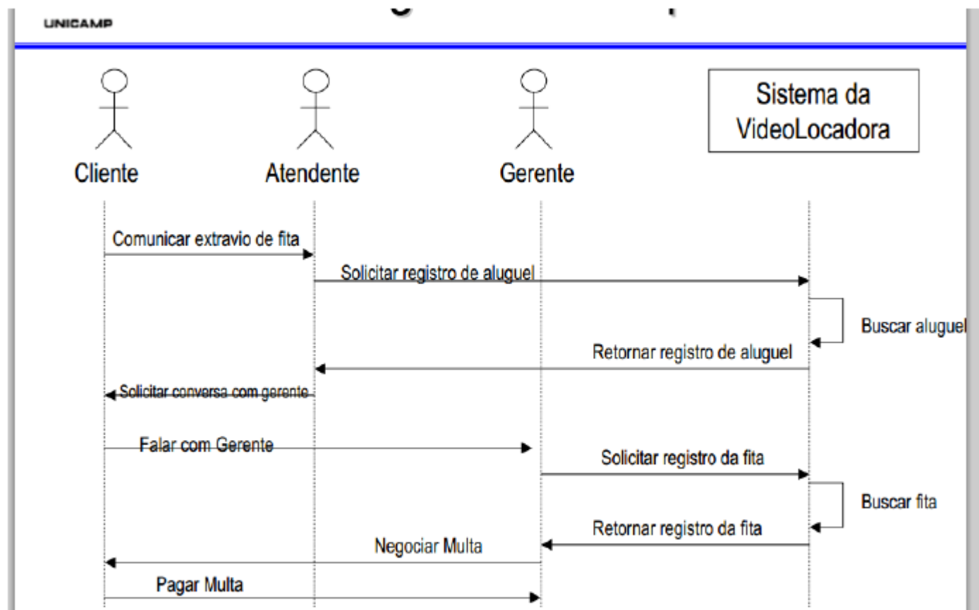
Figura 6: Diagrama de Sequência: Video Locadora
